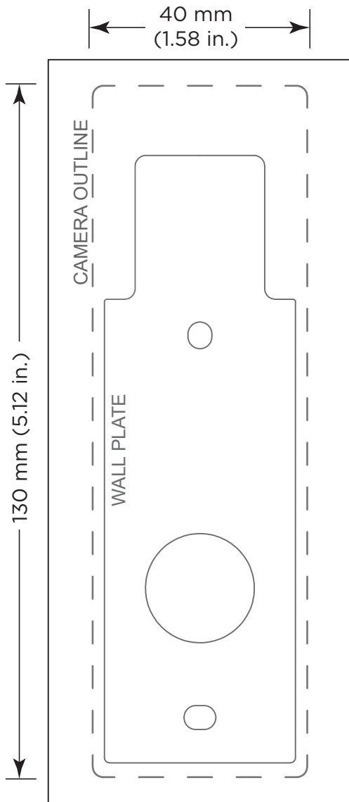
C4-VDB-E (PoE) template
